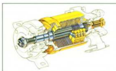
Detail van de viscokoppeling
