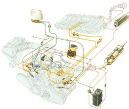
Schema van het Motronic injectie- en ontstekingsysteem
